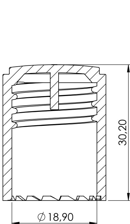
PRZEKRÓJ A-A
