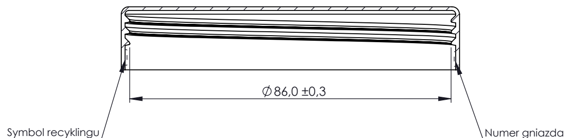
PRZEKRÓJ A-A SKALA 1 : 1
