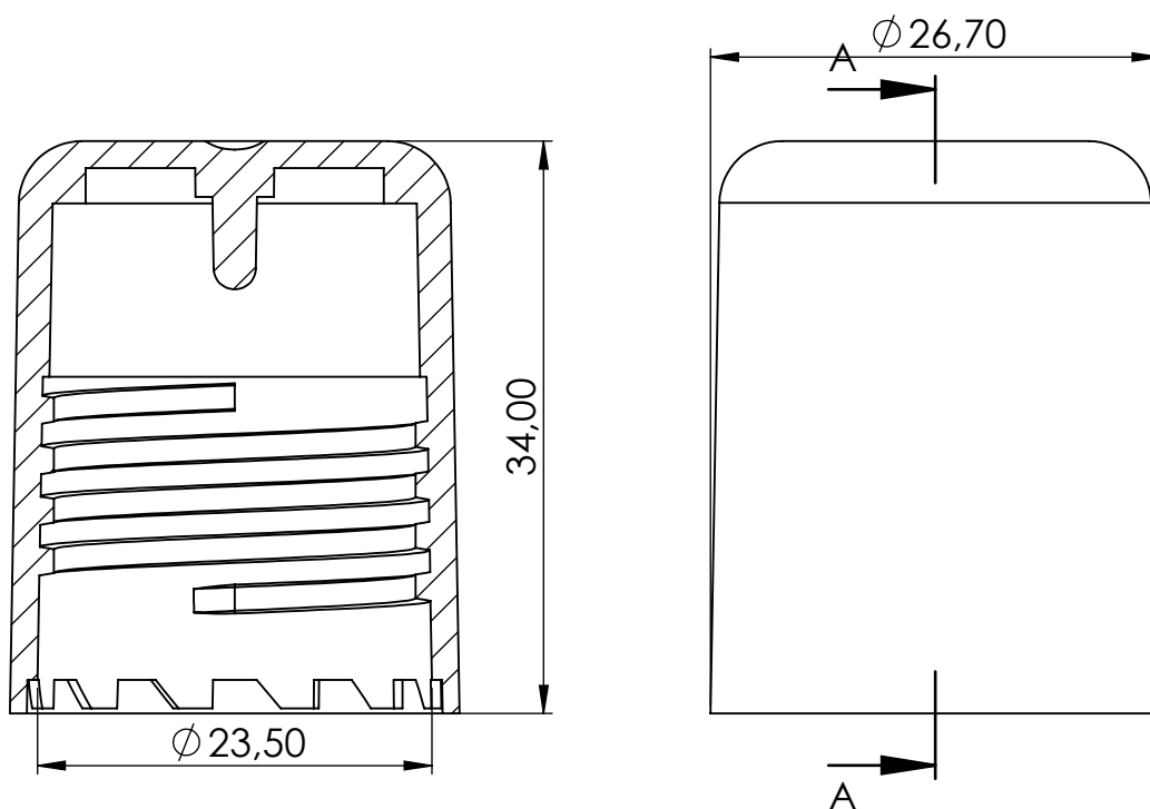
PRZEKRÓJ A-A
