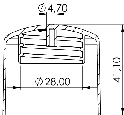
PRZEKRÓJ A-A
