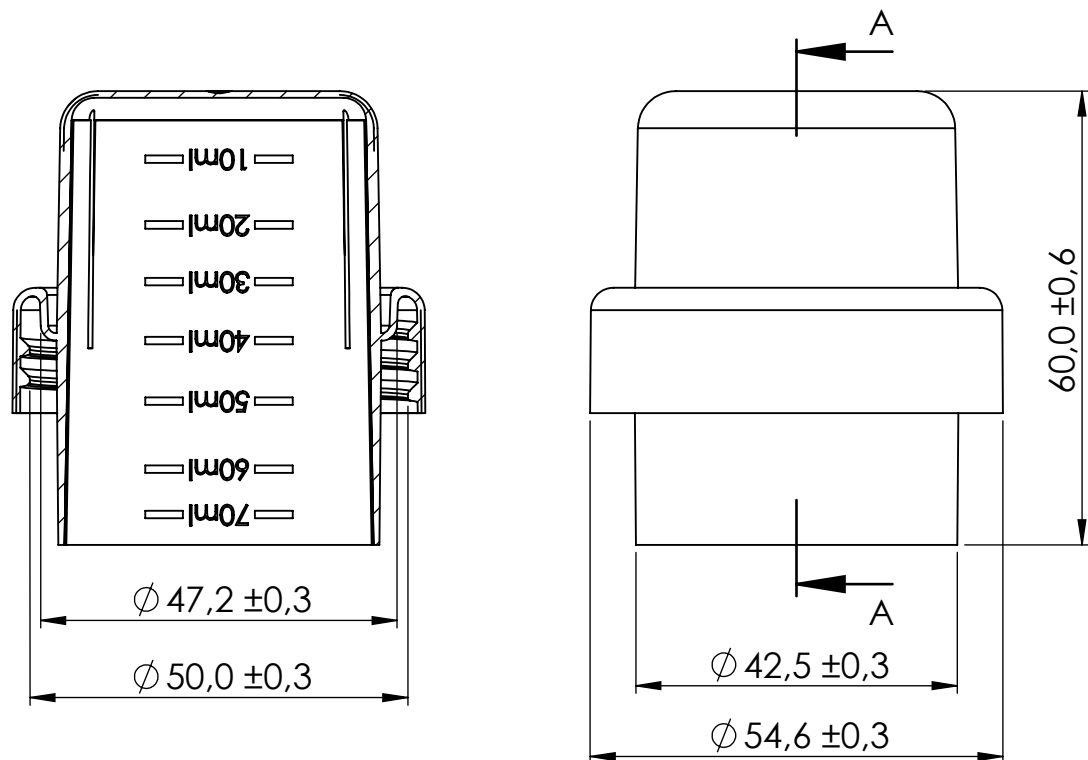
PRZEKRÓJ A-A
